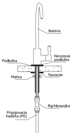
Montáž pomocou rýchlospojky
