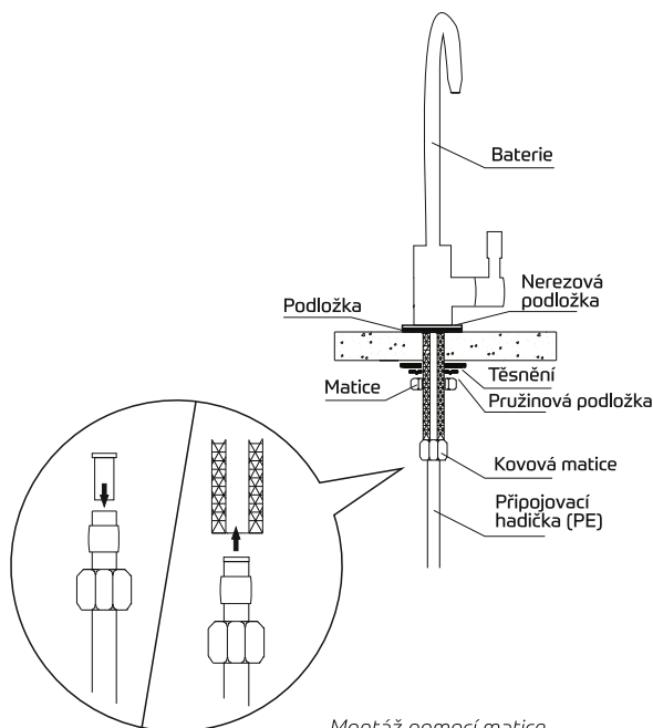
Montáž pomocí matice
