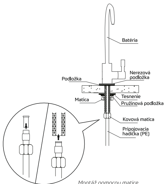
Montáž pomocou matice
