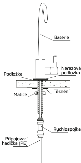
Montáž pomocí rychlospojky
