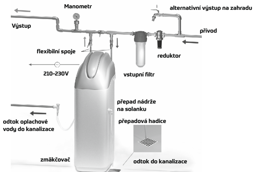
obr.2 Schéma zapojení změkčovače
