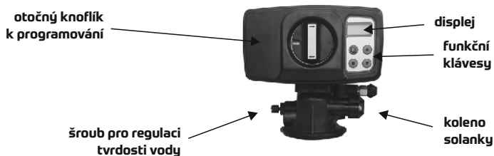
obr.6 Hlavice BNT
