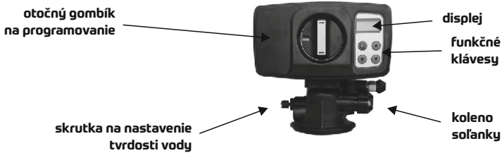
obr.6 Hlava BNT
