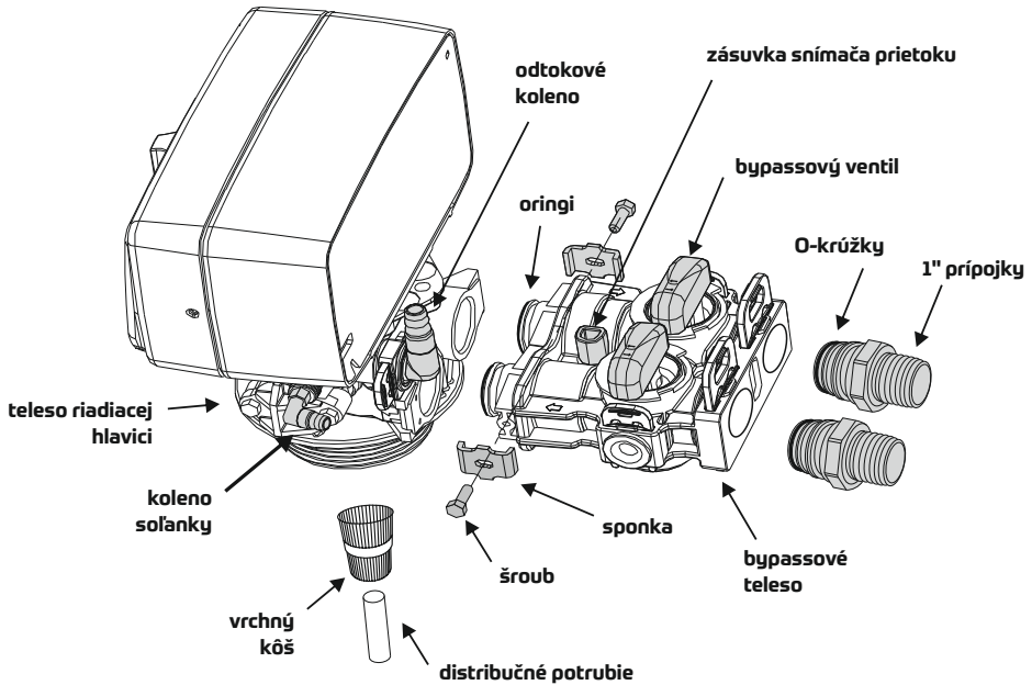
obr.3 Pripojenie bypassu
